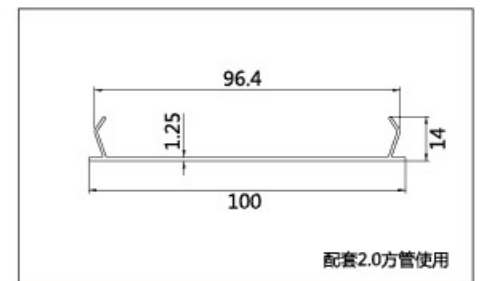
名称: 100FG-G 壁厚: 1.2mm
