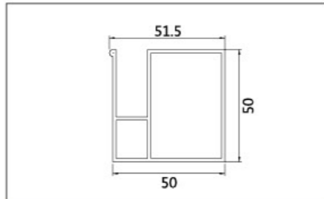
名称: CD-1340 壁厚: 1.5mm
