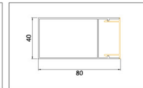
名称: CD-1358 CD-1359 壁厚: 1.1mm 1.1mm
