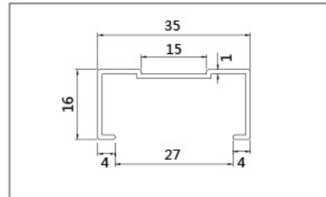
名称: 35x16 加强筋 壁厚: 1.0 1.2 1.4mm
