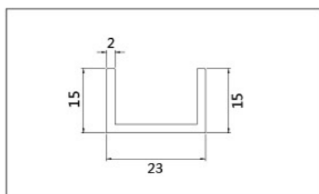
名称: CD-1217 壁厚: 2.0mm
