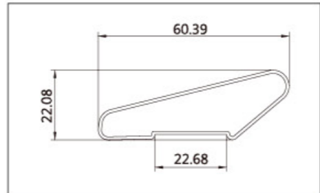
名称: CD-0933 壁厚: 2.0mm
