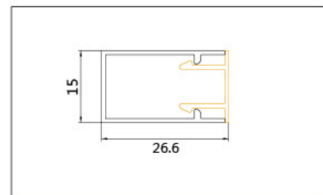
名称: CD-1195 CD-1196 壁厚: 0.8mm 0.8mm
