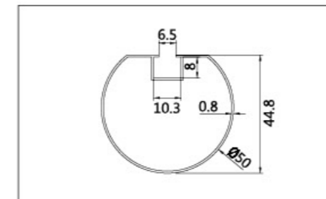
名称: CD-050TH 壁厚: 0.8mm
