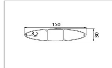
名称: 150x30x1.2 壁厚: 1.2mm
