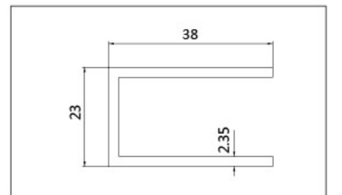
名称: CD-0828 壁厚: 2.35mm
