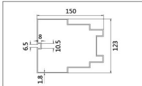
名称: CD-1059 壁厚: 1.8mm
