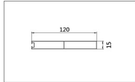
名称：CD-001 壁厚：1.6mm
