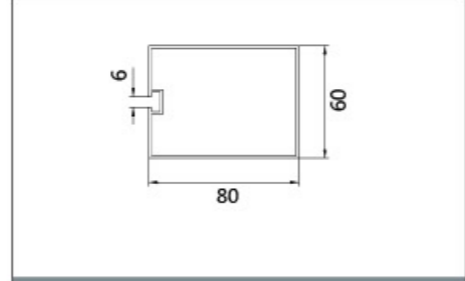
名称: 80x60 壁厚: 1.0 1.2 1.3mm
