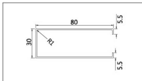
名称: 30x80UC 壁厚: 0.7 0.8 0.9 mm
