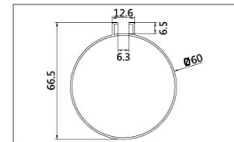
名称: CD-60 壁厚: 0.95mm
