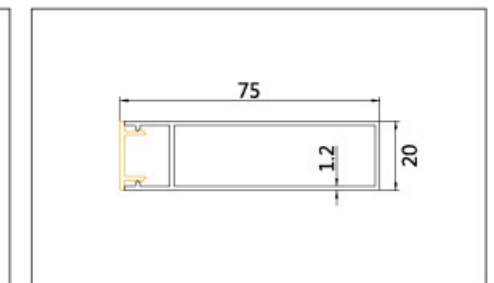
名称: CD-1403 CD-1402 壁厚: 1.2mm 1.2mm
