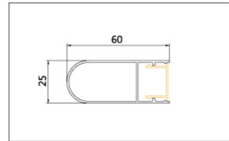
名称: CD-0948 CD-0949 壁厚: 1.2mm 1.0mm
