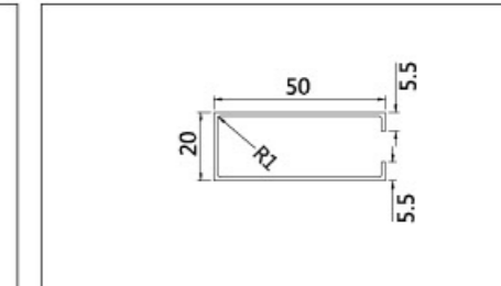
名称: 20x50UC 壁厚: 0.6 0.7 0.9 mm
