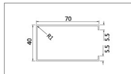
名称: 40x70UC 壁厚: 0.7 0.8 0.9 mm
