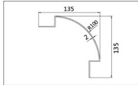
名称: CD-1342 壁厚: 2.0mm
