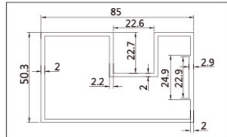
名称: CD-0967 壁厚: 2.0mm
