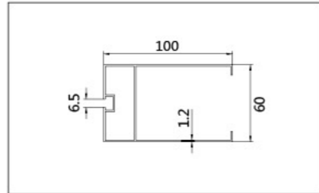
名称: CD-0649 壁厚: 1.2mm
