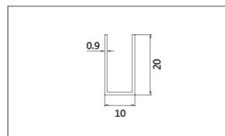
名称: CD-0931 壁厚: 0.9mm
