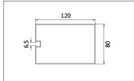
名称: 120x80x1.2TH 壁厚: 1.2 1.4mm
