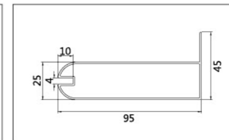
名称: CD-0074 壁厚: 1.1mm
