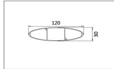
名称: 120x30x1.2 壁厚: 1.2mm
