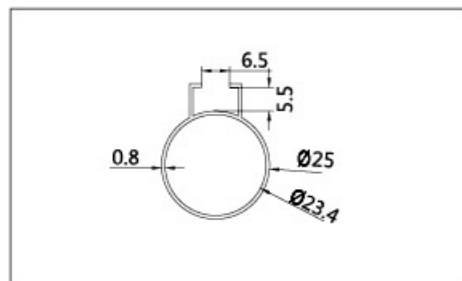
名称: 25YGTH 壁厚: 0.8mm
