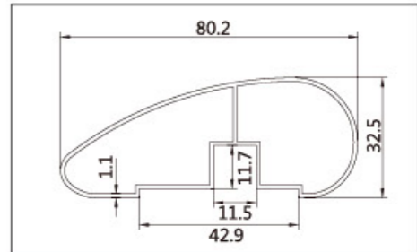
名称: CD-0968 壁厚: 2.0mm
