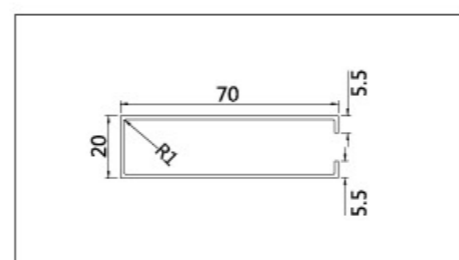
名称: 20x70UC 壁厚: 0.7 0.8 0.9 mm
