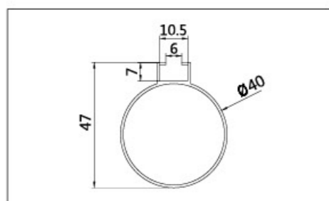
名称: CD-5040 壁厚: 1.0mm
