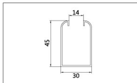
名称: CD-0599 壁厚: 1.2mm
