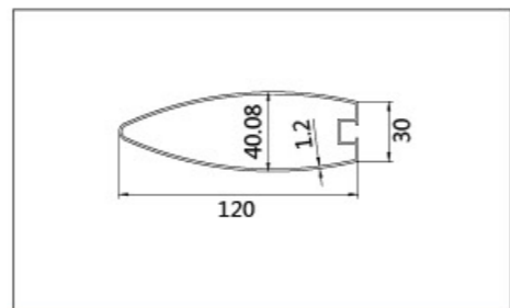
名称：120x40x1.2ZDT 壁厚：1.2mm
